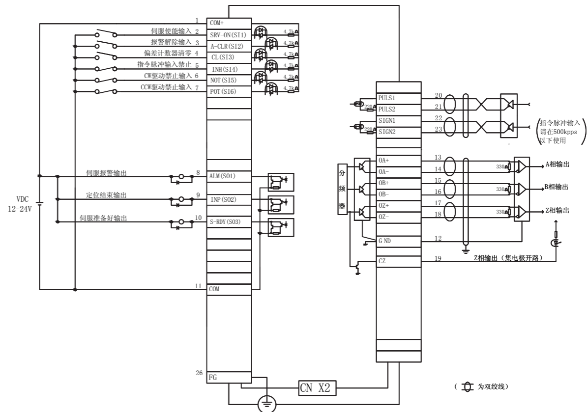
CN X2接线图
